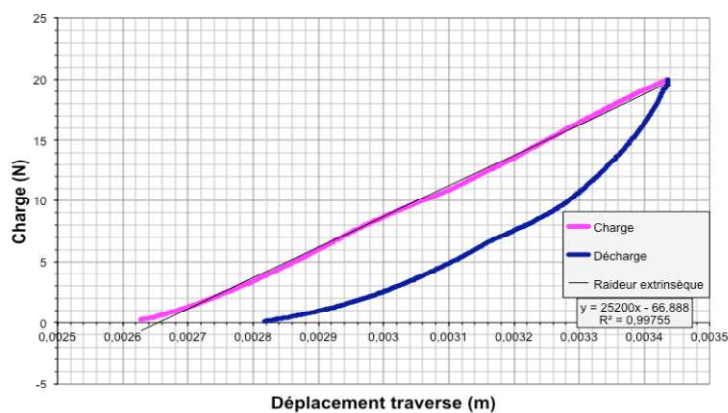
Figure 38 : courbes de charge en fonction de la flèche lors d'essais en flexion 4 points sur un cal osseux
