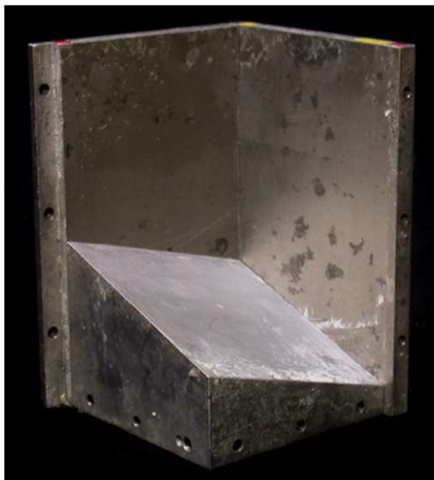
Figure 9: Photographie de la boîte conçue pour un fémur droit. Deux des quatre parois amovibles ont été retirées pour visualiser l'inclinaison du fond de la boîte.
