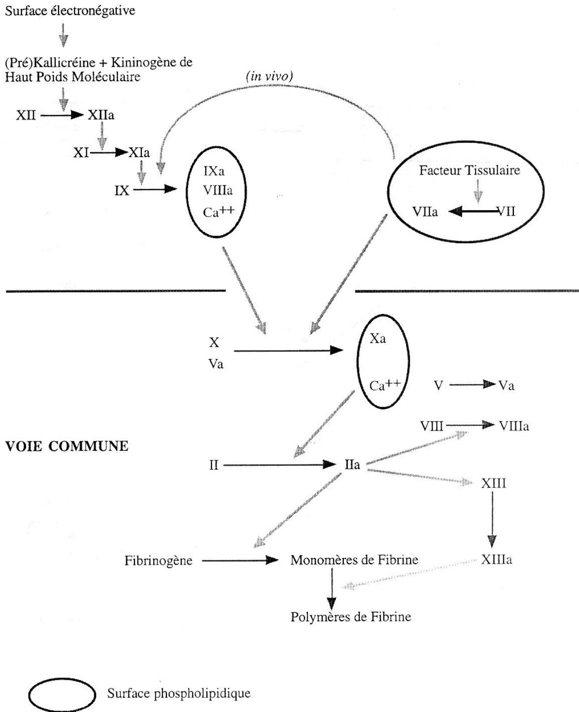
Figure 1 : Schéma simplifié de la coagulation d'après [14]. Les facteurs de la coagulation sont représentés sous-forme de chiffres romains.
