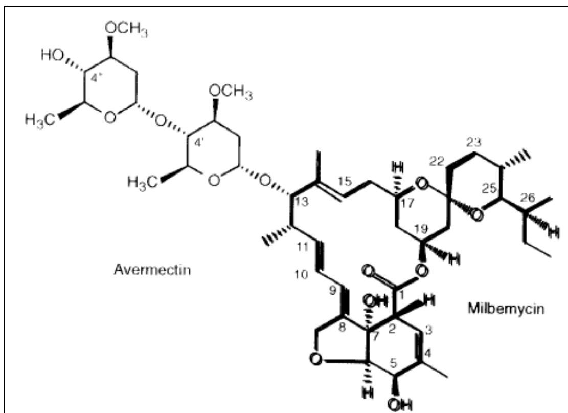
Figure 7 : Superposition des molécules d'ivermectine et de milbémycine. Les molécules représentées ici sont l'ivermectine B 1a et la milbémycine D. La molécule d'ivermectine diffère par la présence d'un groupement disaccharide. Source : Shoop et al, 1995.
