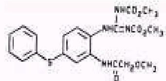
Febentel
